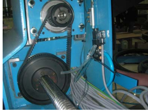
Vidalı mil sait ve döner rulmanlı hareket sistemi
